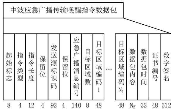
图2 中波应急广播传输唤醒指令数据包通用格式示意图
