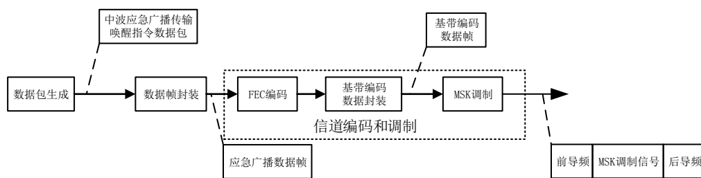
图 6 数据编码和调制流程
