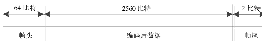
图5 基带编码数据帧格式定义
