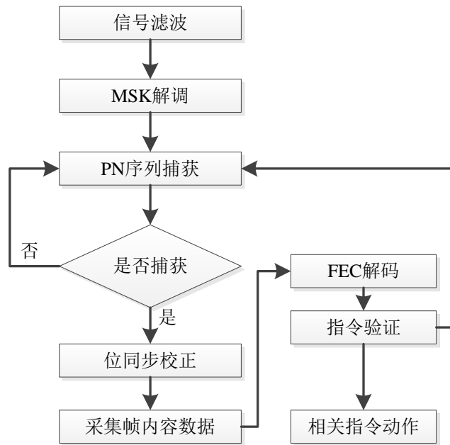
图 D.1 接收装置信号处理流程图
