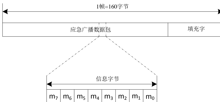
图4 应急广播数据帧格式定义
