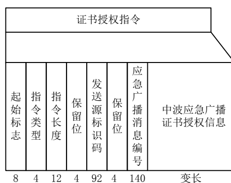
图3 证书授权指令数据包结构图
