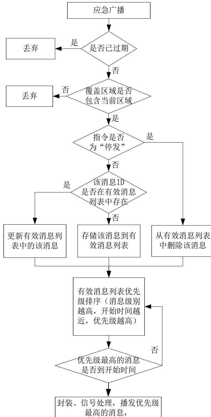
图C. 1 中波发射台应急广播消息接收系统对应急广播消息的处理流程
