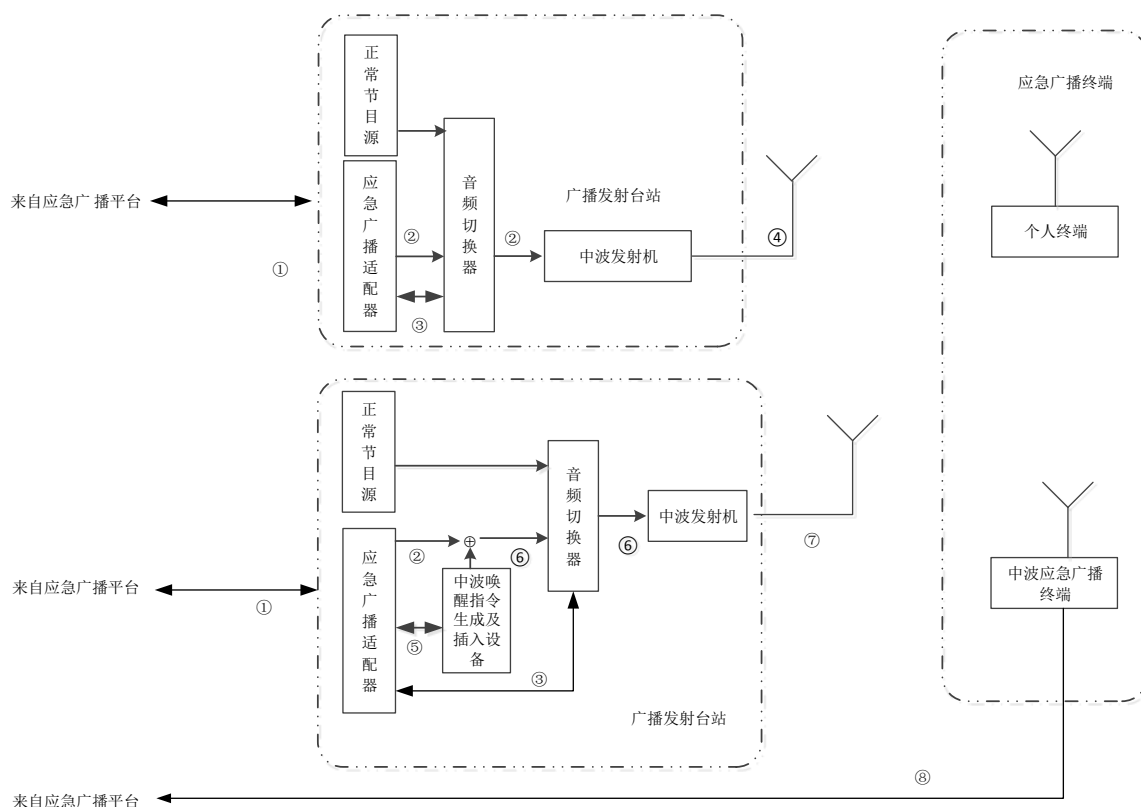
图1 中波调幅广播应急广播系统架构
