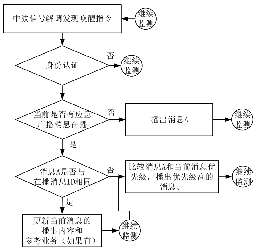
图C.2 中波应急广播接收终端对应急广播消息的处理流程
