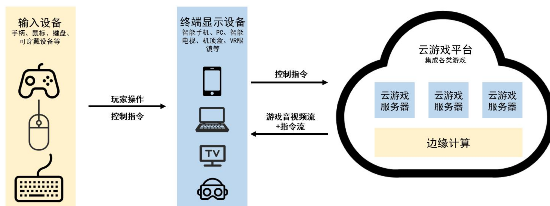
图 1.1 云游戏架构示意图
