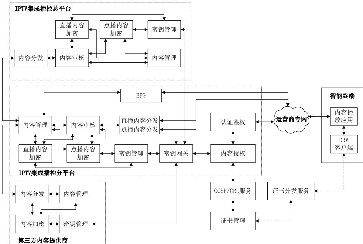
图1 IPTV DRM 系统集成框架
