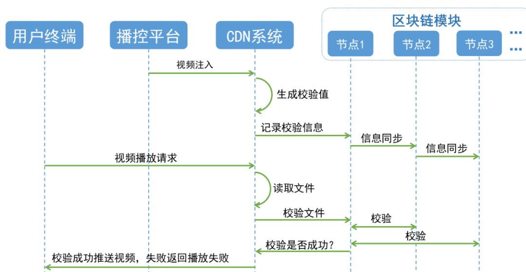
图 3-7 基于区块链的内容校验机制
