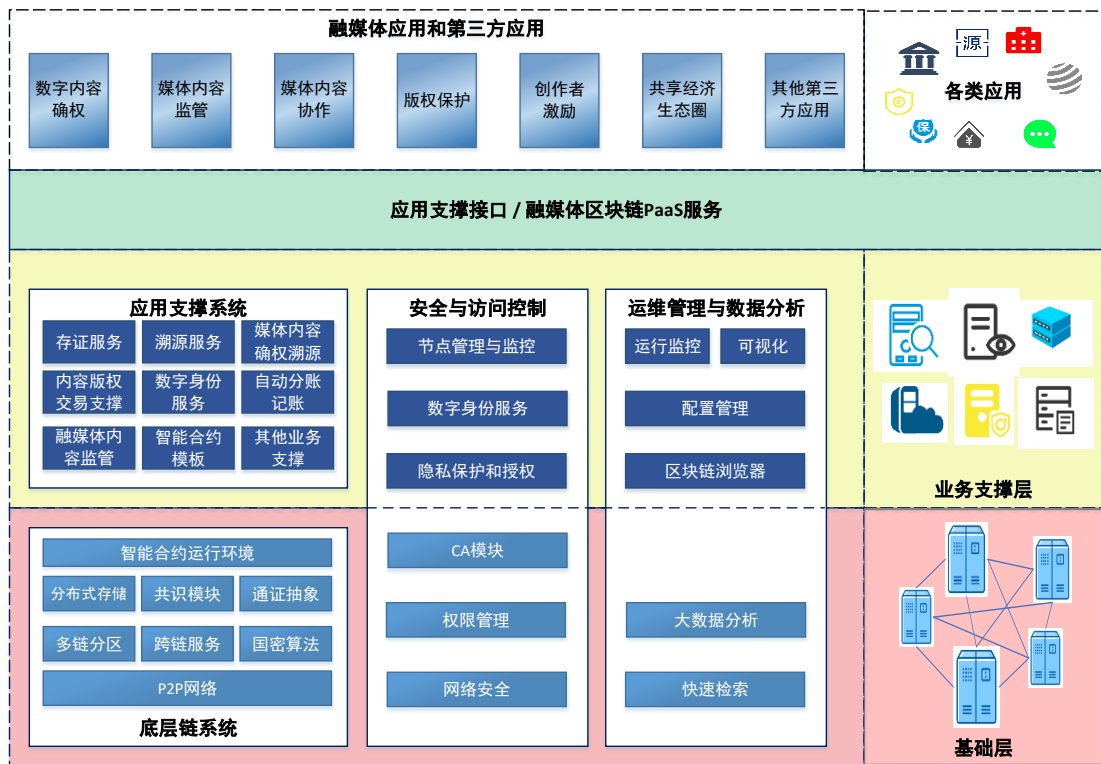
图 A-1 融媒体区块链系统架构
