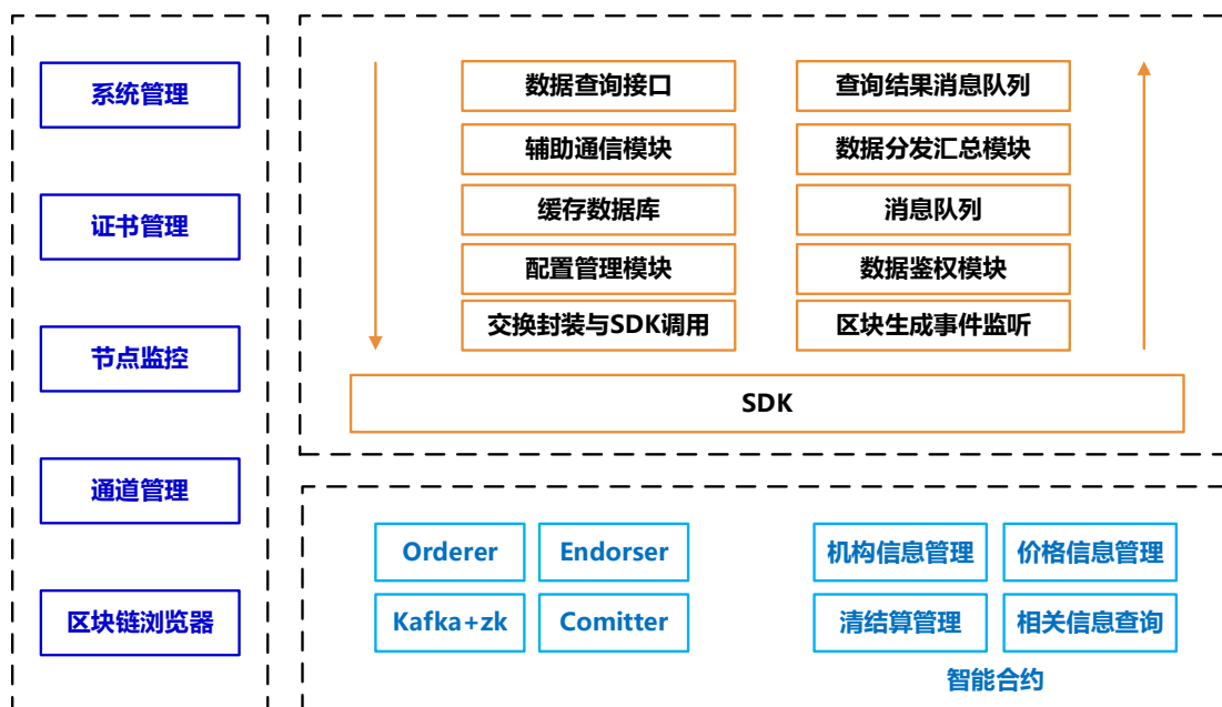
图 A-8 系统结构示意图
