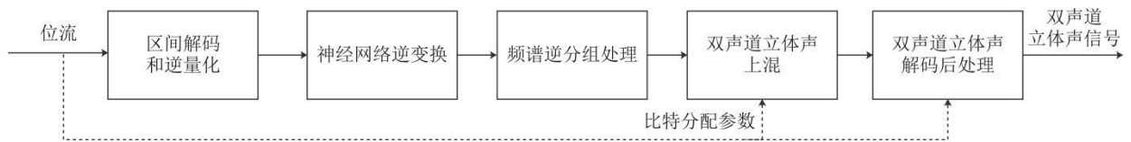
图 6 双声道立体声解码框架
