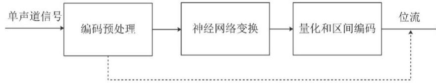
图E.2 通用码率音频单声道编码器
