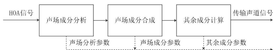
图E.6 通用码率音频 HOA 空间编码
