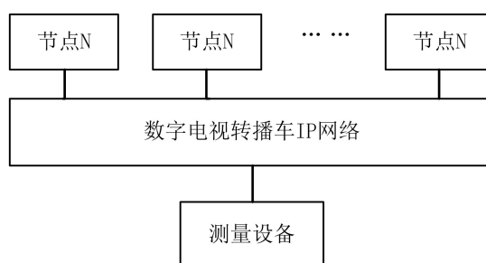
图 20 网络连通性测量框图
