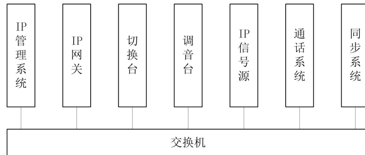
图 8 数字电视转播车典型 IP 通道
