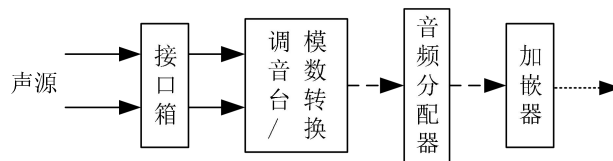
b) 通路 II -模拟输入典型通路
