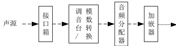
c) 通路 III -数字输入典型通路
