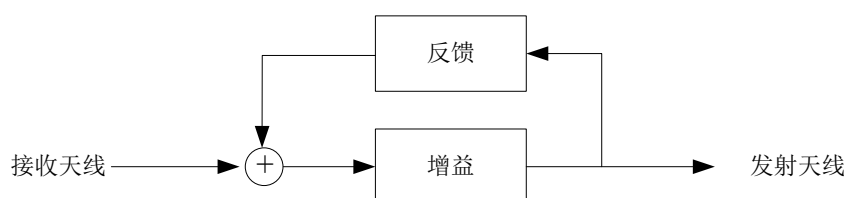
图5 转发器原理
