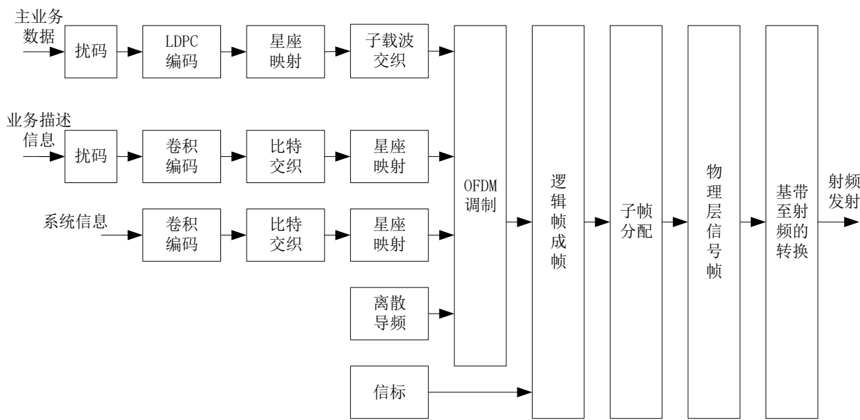
图2 调频频段数字音频广播信道编码和调制子系统的原理框图
