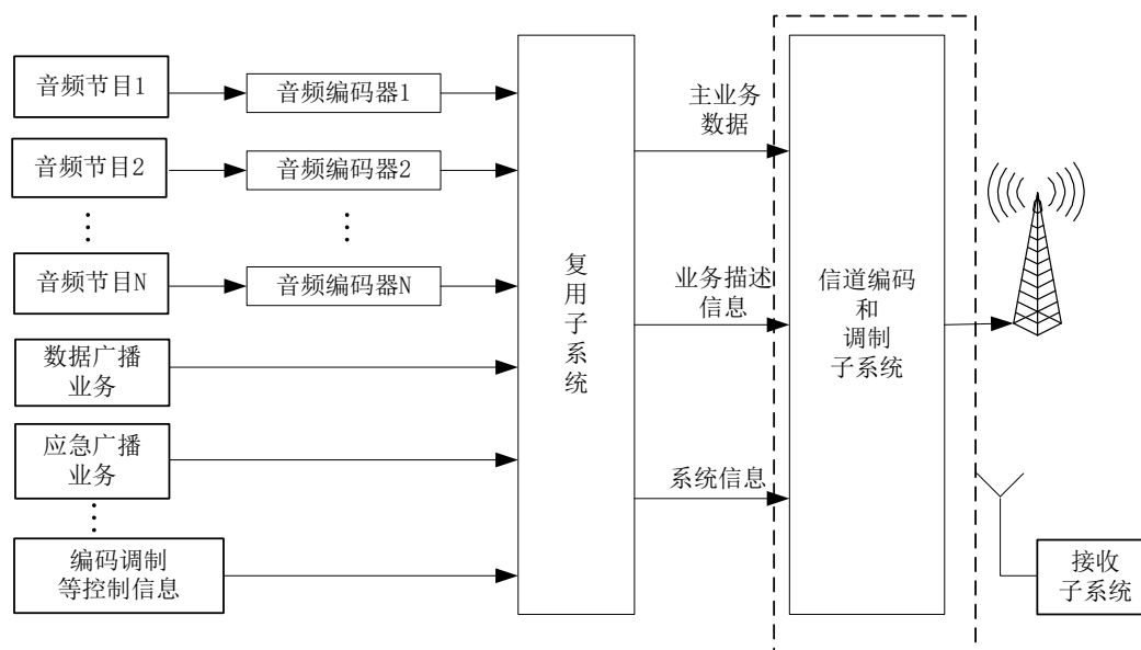
图1 系统结构
