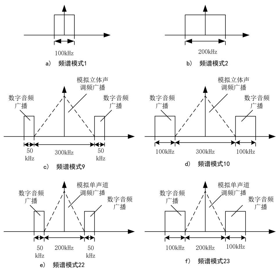
图4 频谱模式
