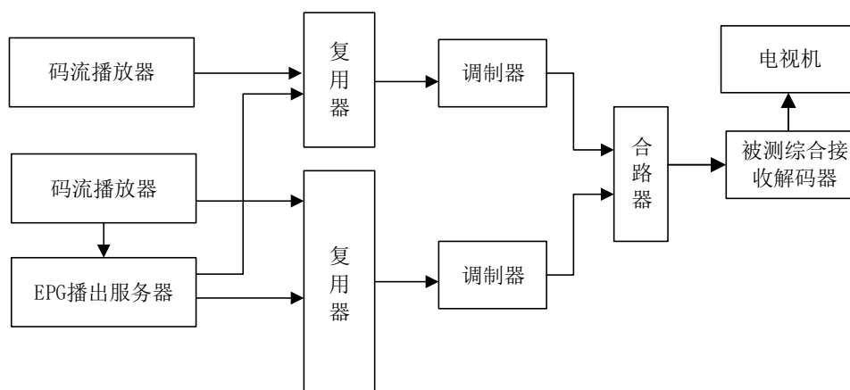
图 F.6 EPG 显示图片测量框图
