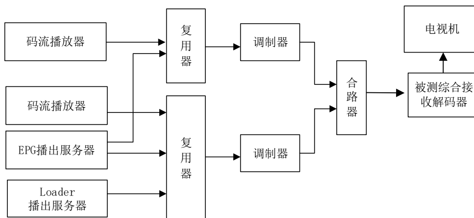
图 6 软件升级测量框图
