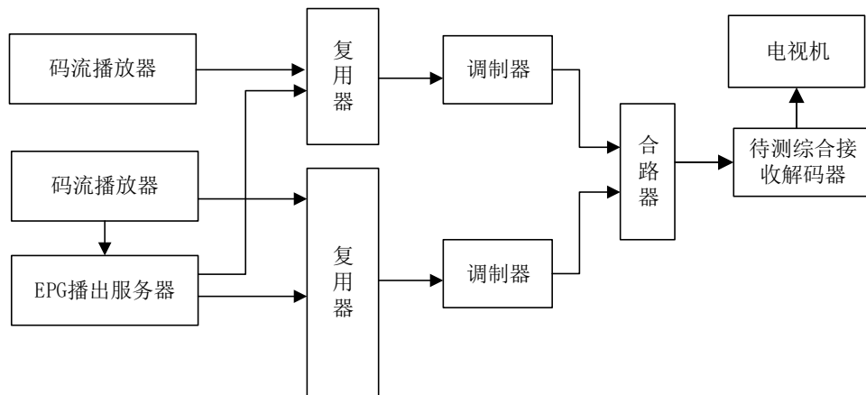
图 G.1 提示信息更新测量框图
